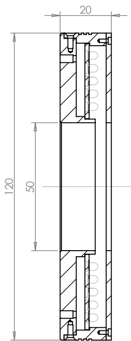
剖面 A-A
